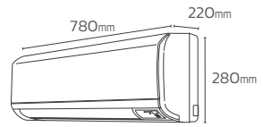
RPK-1.8-2.3FSNQ5 12.5kg
